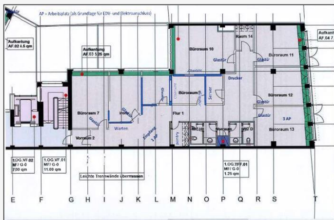
Grundriss
