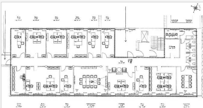
Grundriss
